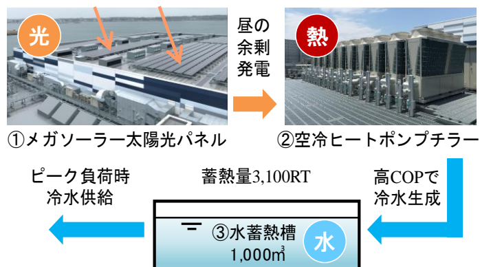
図 太陽光余剰電力の蓄熱槽利用
