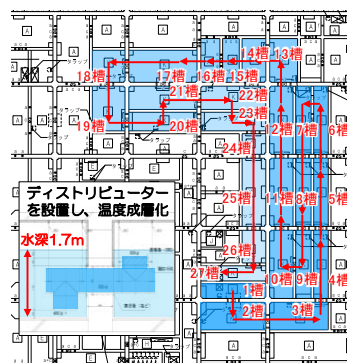
図 低層連結型蓄熱槽
