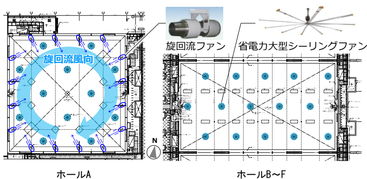
図 シーリングファン・旋回流ファン配置
