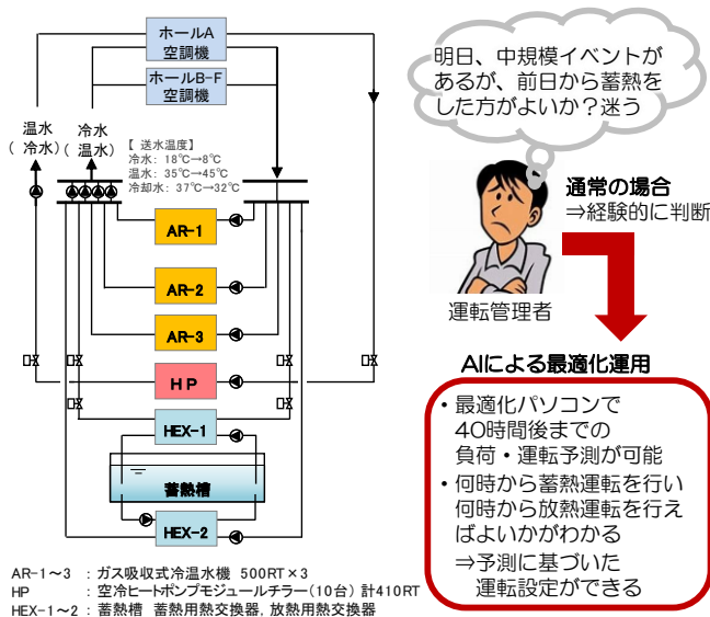
図 熱源システムと AI による最適化運用
